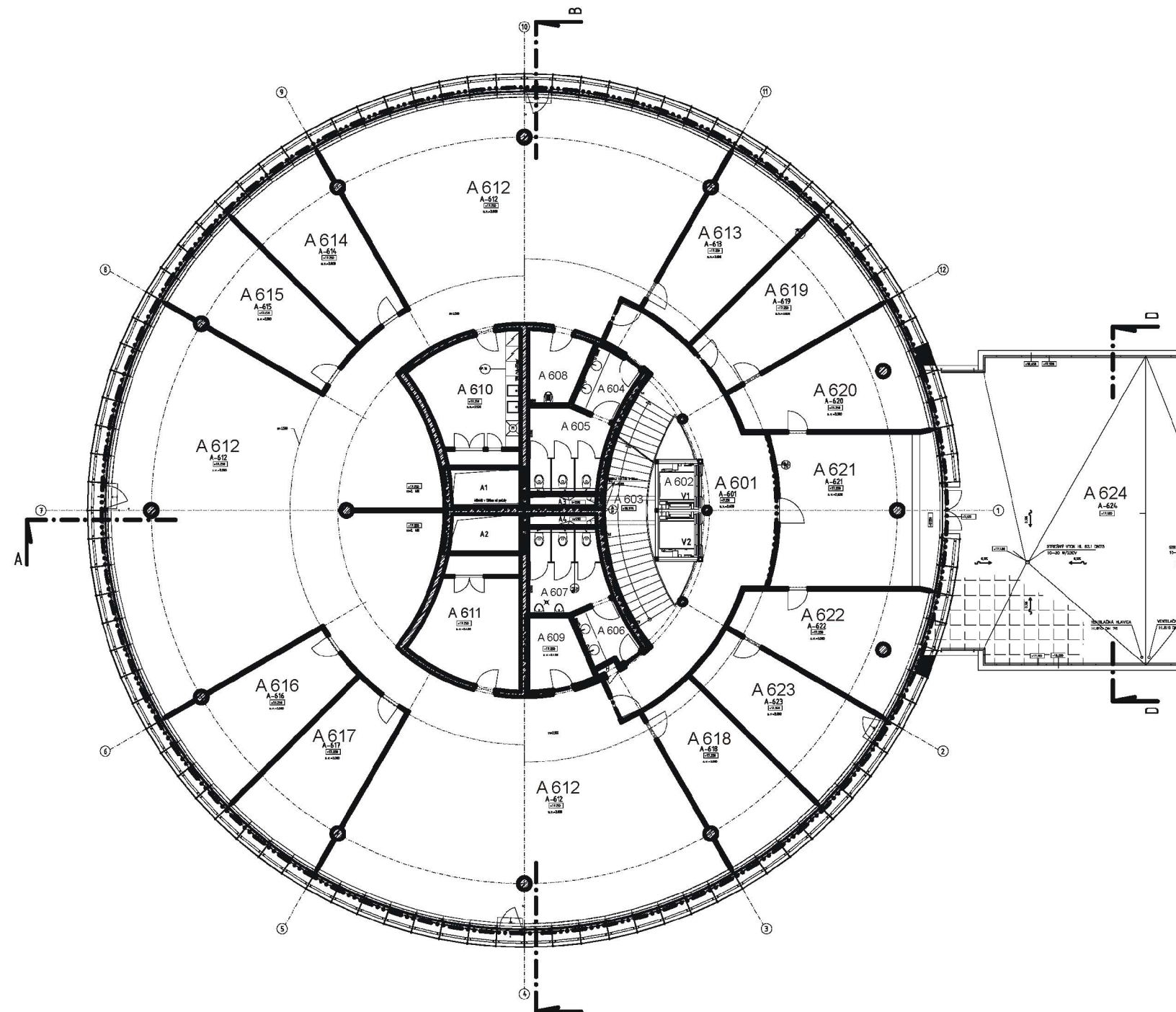
časť A objektu SO 01
